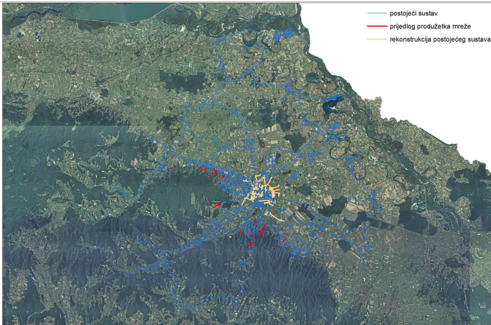
Slika 2-5a. Postojeći i planirani dijelovi sustava vodoopskrbe
