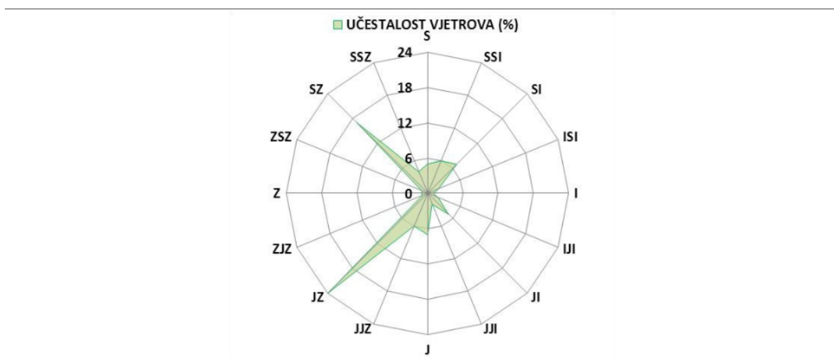
Slika 3-19. Ruža vjetrova za područje Grada Koprivnica
