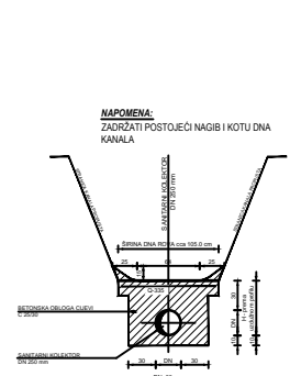
POPREČNI PRESJEK ROVA PO ODVODNOM KANALU PRIJE PROPUSTA - Kolektor K-2 - od stac. 0+095,14 m do stac. 0+140,42 m
