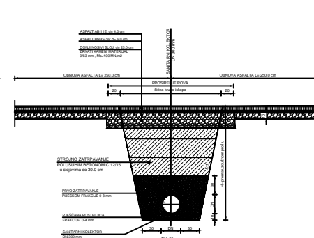
POPREČNI PRESJEK ROVA KOD PREKOPA PROMETNICE - DRŽAVNA CESTA -
