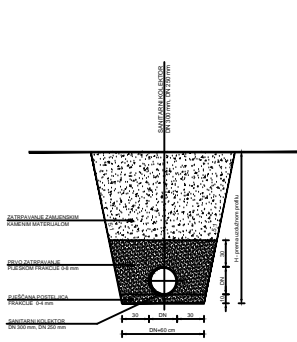
POPREČNI PRESJEK ROVA PROJEKTIRANOG SANITARNOG KOLEKTORA - ZEMLJANE POVRŠINE -
