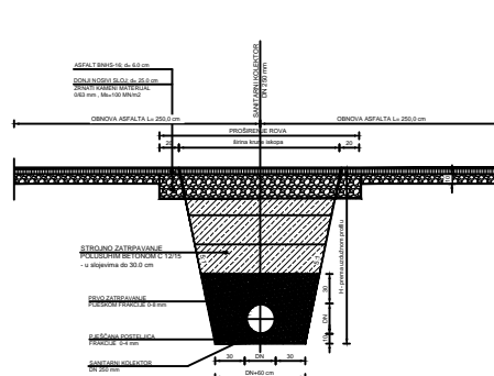
POPREČNI PRESJEK ROVA KOD PREKOPA PROMETNICE - LOKALNE CESTE -
