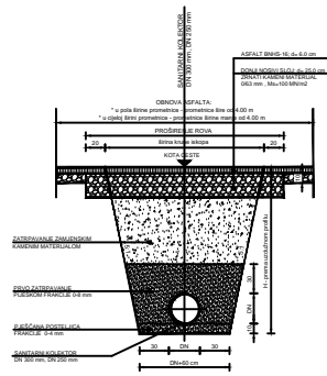
POPREČNI PRESJEK ROVA PROJEKTIRANOG SANITARNOG KOLEKTORA - LOKALNE CESTE -
