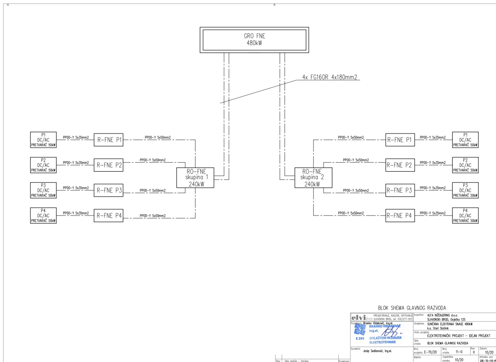
Slika 4. Blok shema glavnog razvoda (Izvor: Idejni elektrotehnički projekt, oznake E-70/20, Elvi d.o.o., Slavonski Brod, listopad 2020. godine)
