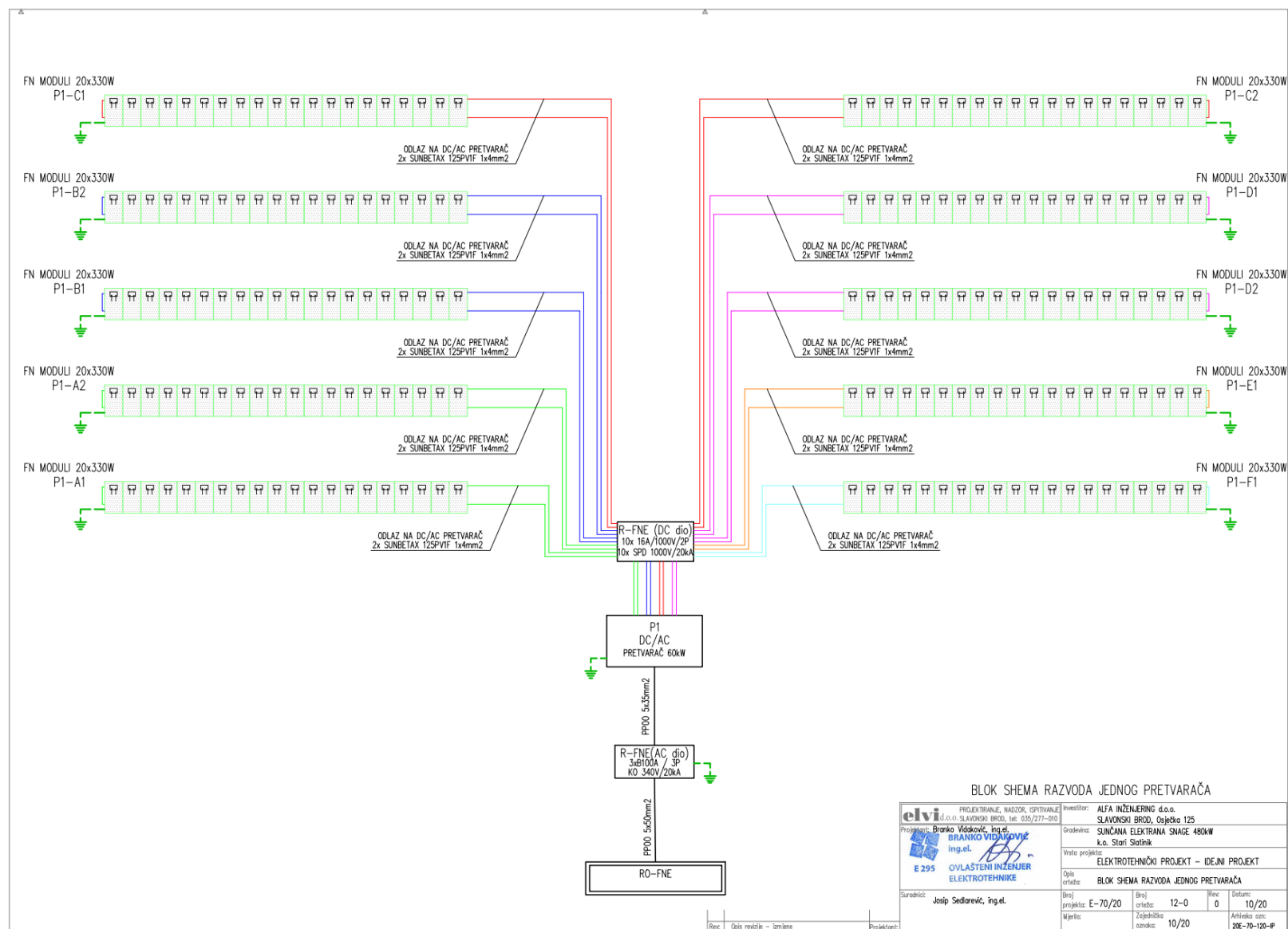
Slika 5. Blok shema spajanja izmjenjivača (Izvor: Idejni elektrotehnički projekt, oznake E-70/20, Elvi d.o.o., Slavonski Brod, listopad 2020. godine)
