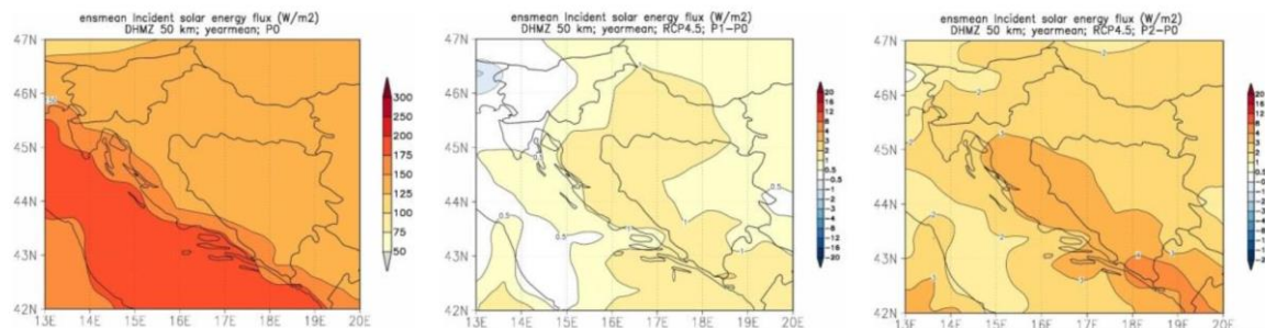
Slika 22. Srednji godišnji fluks ulazne sunčane energije ( W/m^2 ) u srednjaku ansambla iz četiri integracije RegCM modelom. Lijevo: referentno razdoblje 1971.-2000.; sredina: promjena u razdoblju 2011.-2040; desno: promjena u razdoblju 2041.-2070.
