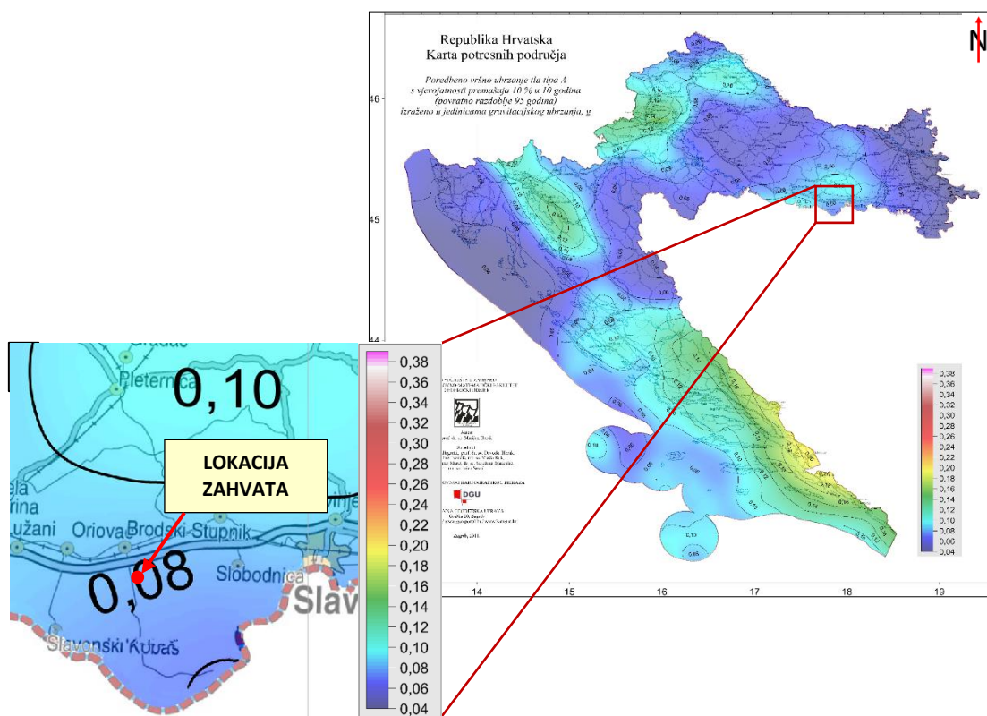
Slika 8. Isječak iz Karte potresnih područja Republike Hrvatske za povratno razdoblje od 95 godina na kojem je vidljiva lokacija zahvata
