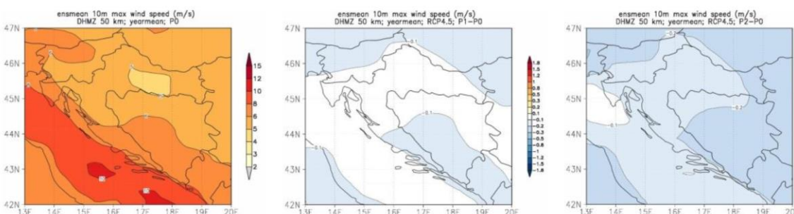
Slika 20. Srednja godišnja maksimalna brzina vjetra (m/s) u srednjaku ansambla iz četiri integracije RegCM modelom. Lijevo: referentno razdoblje 1971.-2000.; sredina: promjena u razdoblju 2011.-2040.; desno: promjena u razdoblju 2041.-2070.
