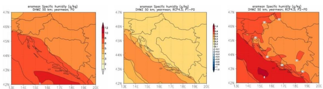
Slika 23. Srednja godišnja specifična vlažnost zraka (g/kg) u srednjaku ansambla iz četiri integracije RegCM modelom. Lijevo: referentno razdoblje 1971.-2000.; sredina: promjena u razdoblju 2011.-2040.; desno: promjena u razdoblju 2041.-2070.
