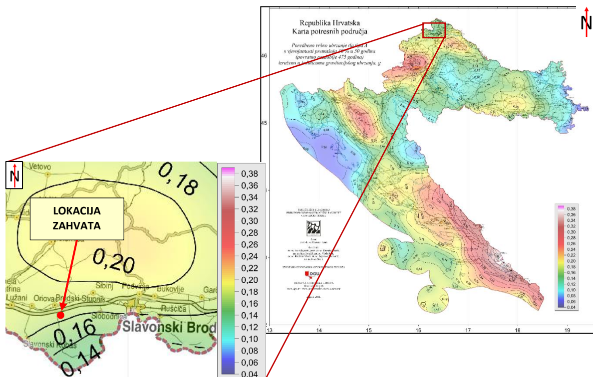
Slika 9. Isječak iz Karte potresnih područja Republike Hrvatske za povratno razdoblje od 475 godina na kojem je vidljiva lokacija zahvata
