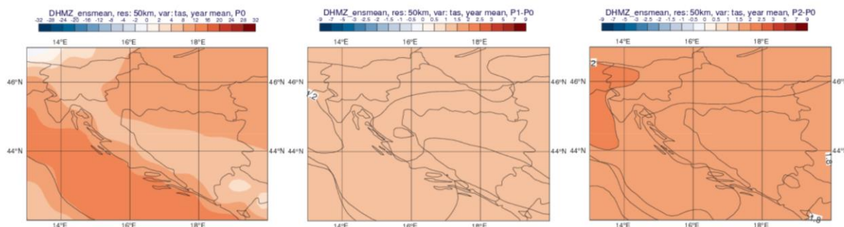
Slika 14. Srednja godišnja temperatura zraka (°C) u srednjaku ansambla iz četiri integracije RegCM modelom. Lijevo: referentno razdoblje 1971.-2000.; sredina: promjena u razdoblju 2011.-2040.; desno: promjena u razdoblju 2041.-2070.
