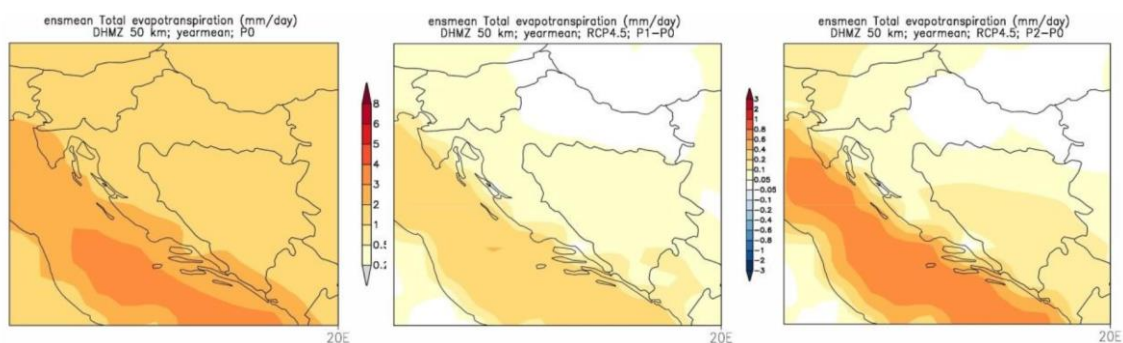
Slika 18. Godišnja evapotranspiracija (mm/dan) u srednjaku ansambla iz četiri integracije RegCM modelom. Lijevo: referentno razdoblje 1971.-2000.; sredina: promjena u razdoblju 2011.-2040.; desno: promjena u razdoblju 2041.-2070.
