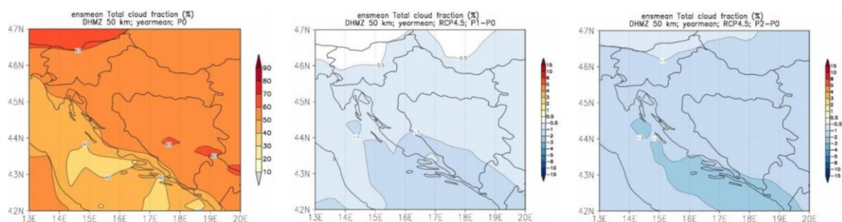
Slika 21. Srednja godišnja ukupna naoblaka (%) u srednjaku ansambla iz četiri integracije RegCM modelom. Lijevo: referentno razdoblje 1971.-2000.; sredina: promjena u razdoblju 2011.-2040.; desno: promjena u razdoblju 2041.-2070
