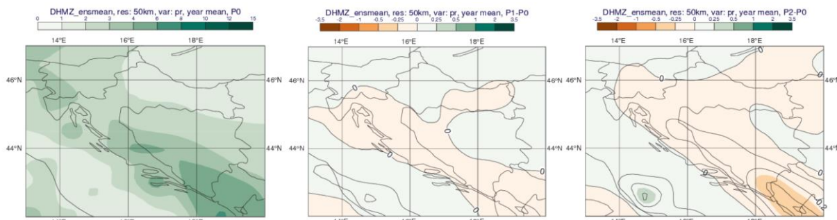
Slika 17. Ukupna godišnja količina oborine (mm/dan) u srednjaku ansambla iz četiri integracije RegCM modelom. Lijevo: referentno razdoblje 1971.-2000.; sredina: promjena u razdoblju 2011.-2040.; desno: promjena u razdoblju 2041-2070.
