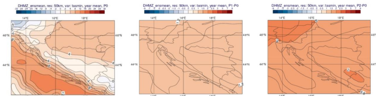
Slika 16. Srednja godišnja minimalna temperatura zraka (°C) u srednjaku ansambla iz četiri integracije RegCM modelom. Lijevo: referentno razdoblje 1971.-2000.; sredina: promjena u razdoblju 2011.-2040.; desno: promjena u razdoblju 2041.-2070.
