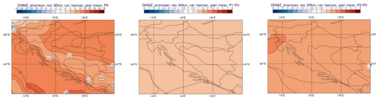
Slika 15. Srednja godišnja maksimalna temperatura zraka (°C) u srednjaku ansambla iz četiri integracije RegCM modelom. Lijevo: referentno razdoblje 1971.-2000.; sredina: promjena u razdoblju 2011.-2040.; desno: promjena u razdoblju 2041.-2070.
