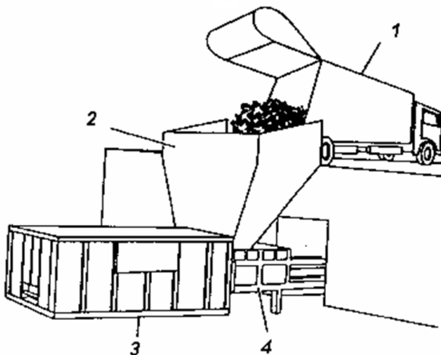
Slika 1./3. Objekt za pretovar otpada (izuzev glomaznog otpada) sistemom izravnog istovara otpada u lijevak opremljena stacionarnim sabijačem: 1- kamion smećar; 2 - lijevak; 3 - kontejner velikog kapaciteta; 4 - sabijač (preša, kompaktor) [2]
