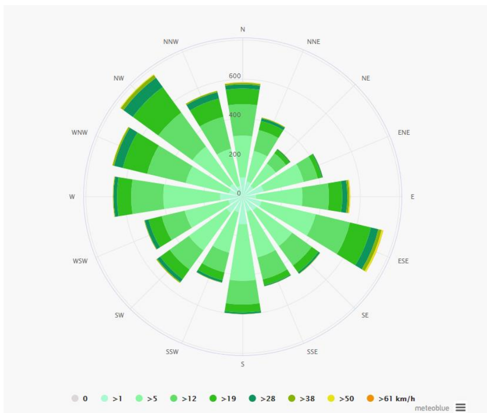
Slika 2./13. Ruža vjetrova za područje Stari Jankovci [13]
