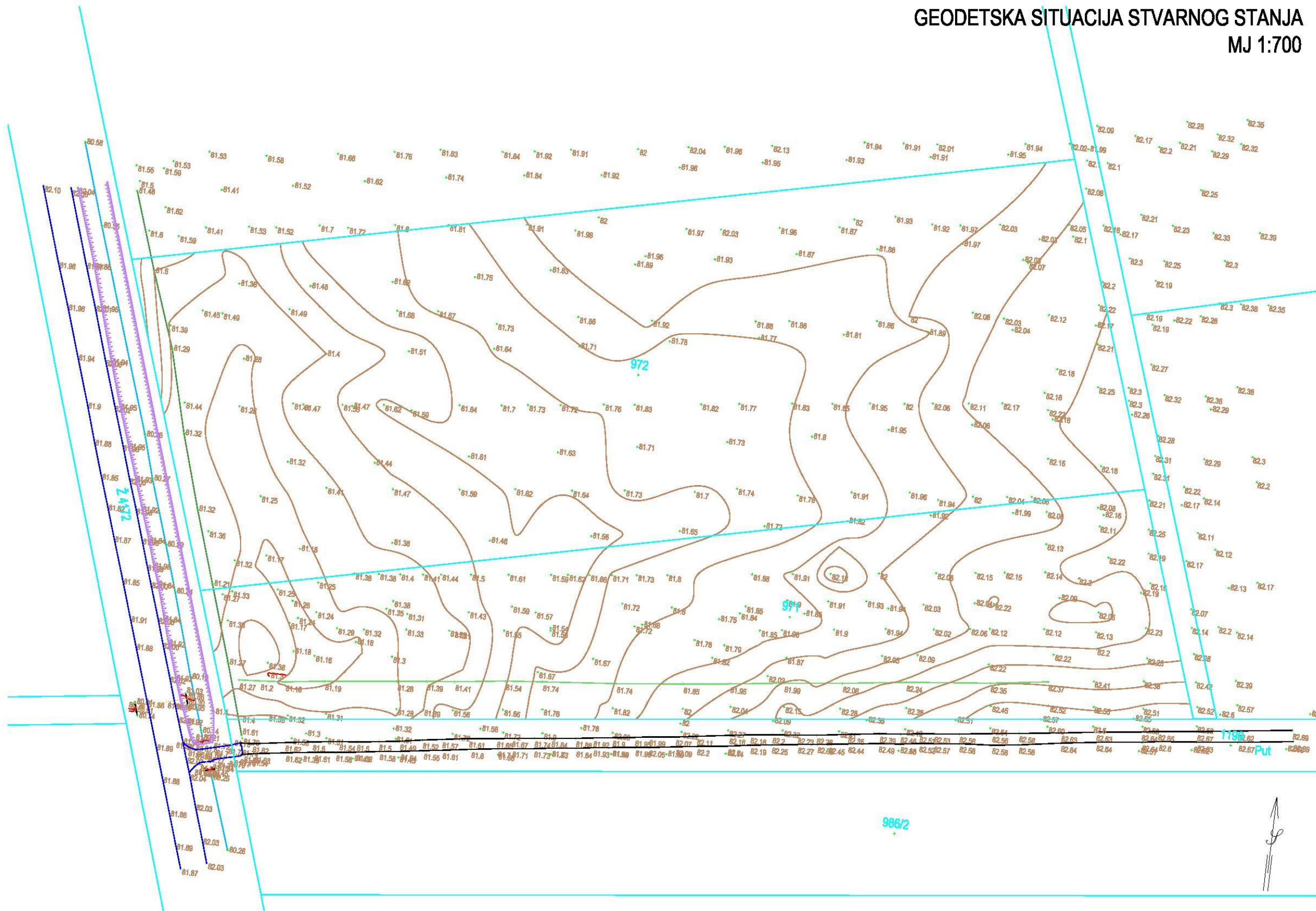
Slika 1./4. Geodetski situacijski nacrt stvarnog stanja [1]
