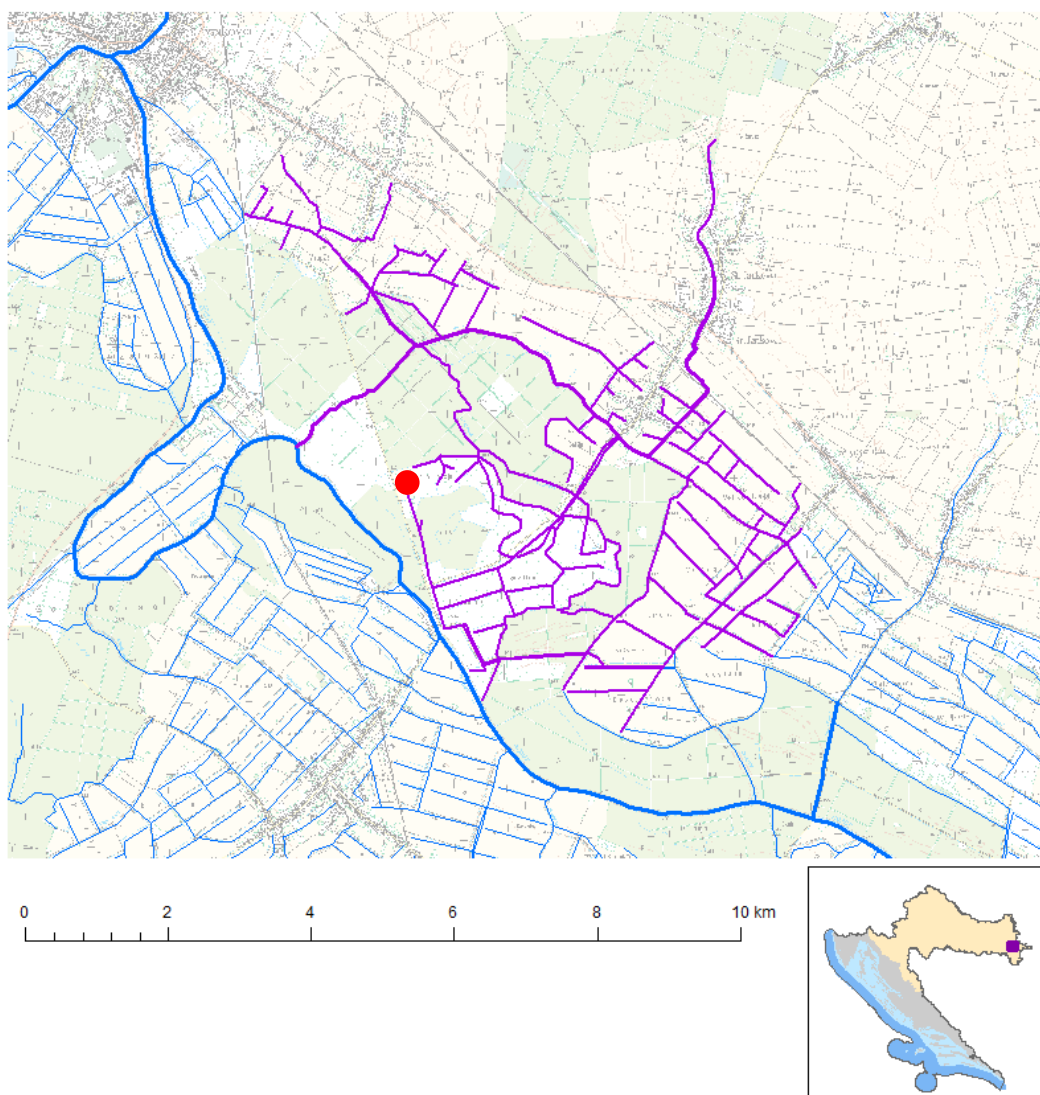
Slika 2./8. Karta vodnog tijela CSRN0201_001, Vidor [10]
