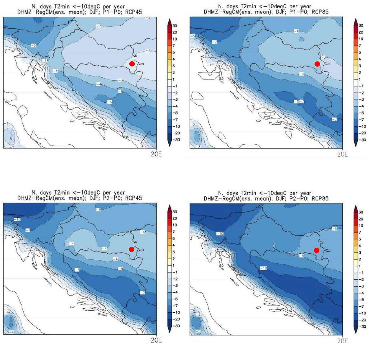
Slika 2./17. Promjene srednjeg broja ledenih dana (dan kada je minimalna temperatura manja ili jednaka -10^{\circ}\text{C} ) u odnosu na referentno razdoblje 1971.-2000. u srednjaku ansambla iz četiri integracije RegCM modelom. Lijevo: scenarij RCP4.5; desno: scenarij RCP8.5. Prvi red: promjene u razdoblju 2011.-2040. godine; drugi red: promjene u razdoblju 2041.-2070. godine. Mjerna jedinica: broj događaja u godini. Sezona: zima. [14]
