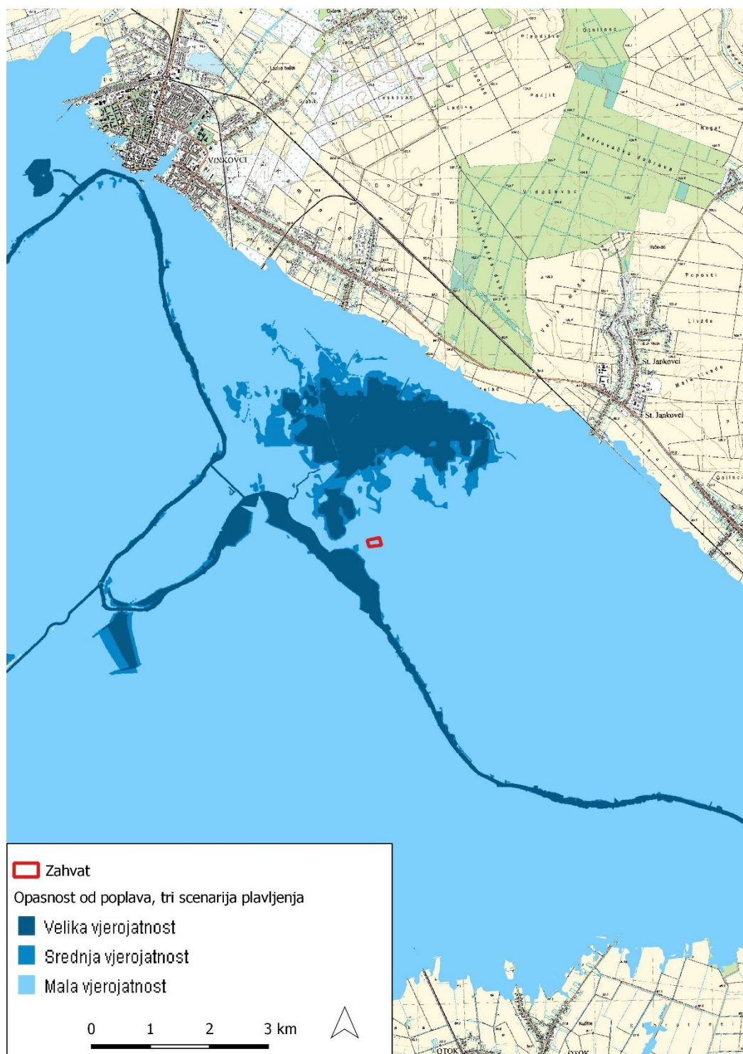
Slika 2./9. Vjerojatnost poplavljanja na širem području lokacije zahvata [11]
