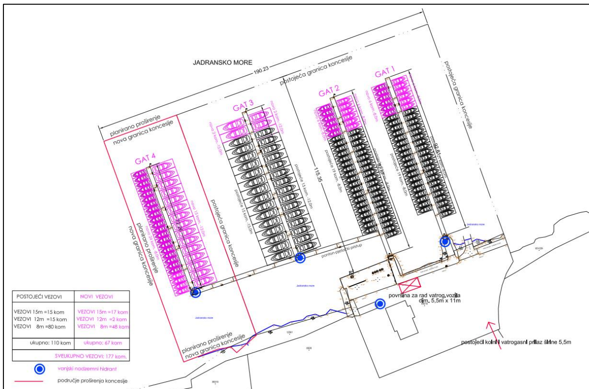
Slika 4. Planirano stanje: situacija – mjere zaštite od požara
