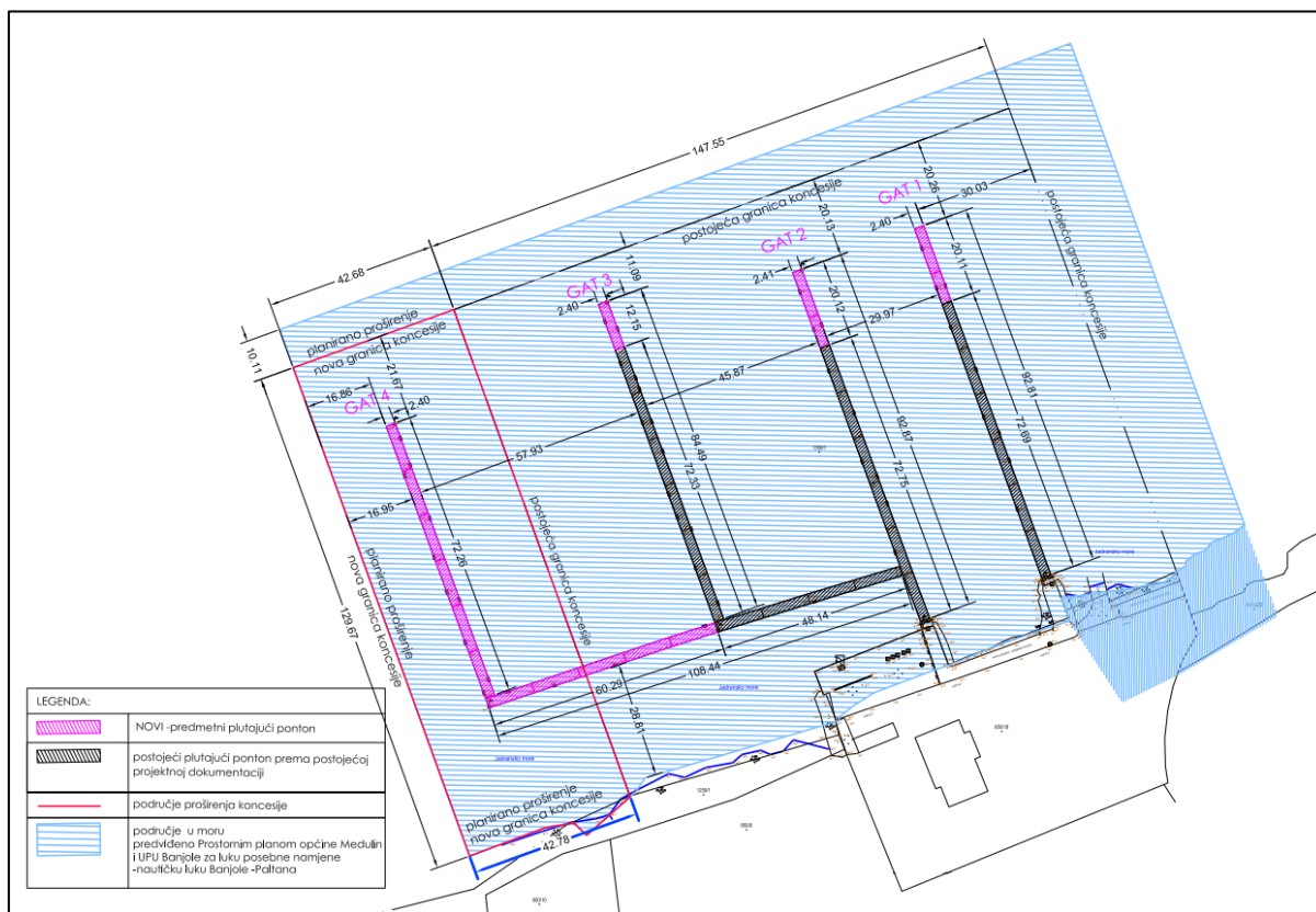
Slika 2. Planirano stanje: situacija – plutajući pontoni
